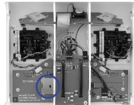
SD-kaartsleuf in de radio
